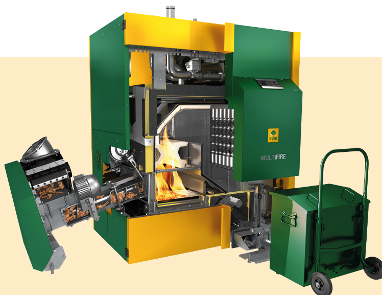
Multifire / Pelletfire Chaudière à plaquettes 20-120 kW à granulés 45-135 kW TDS 150-300 kW
